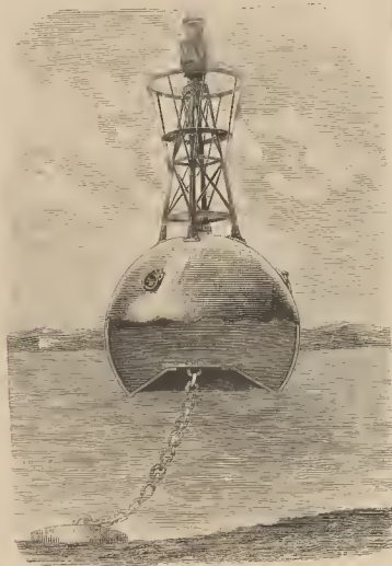
Fig. 4. Boya luminosa anclada en el mar
